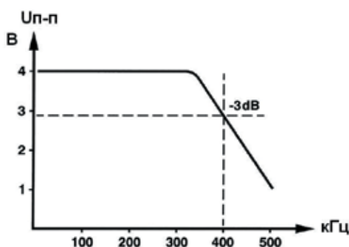
Увеличение частотного диапазона до 400 кГц в моделях АК ИП-1106 (сигналы малых уровней – до 4 Впик-пик)
