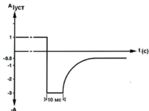
Формирование 3 кратного выходного тока t=10 мс обратной полярности для разряда нагрузки при установке опции TOE 8810/107
