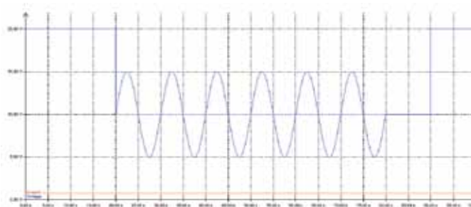
Редактирование Uвых сигнала произвольной формы (окно ПО ArbNet)
