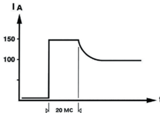
Увеличение амплитуды импульсного выходного тока нагрузки 1,5 x I_{уст} для АКПП-1107А-40-100 ( t_{имп.} \sim 20 мс)
