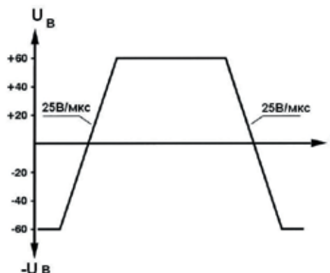
Скорость смены полярности для АК ИП-1106-60-2,5 (в полном диапазоне Uвых)
