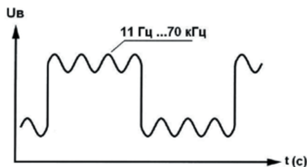
Формирование пульсаций бортовой сети ТС (ripple) с помощью опции TOE 8810/107
